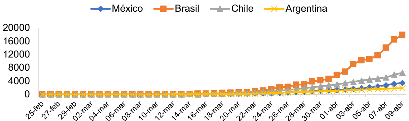
Gráfico 1. Número de casos confirmados por contagio de COVID-19 en países seleccionados.
